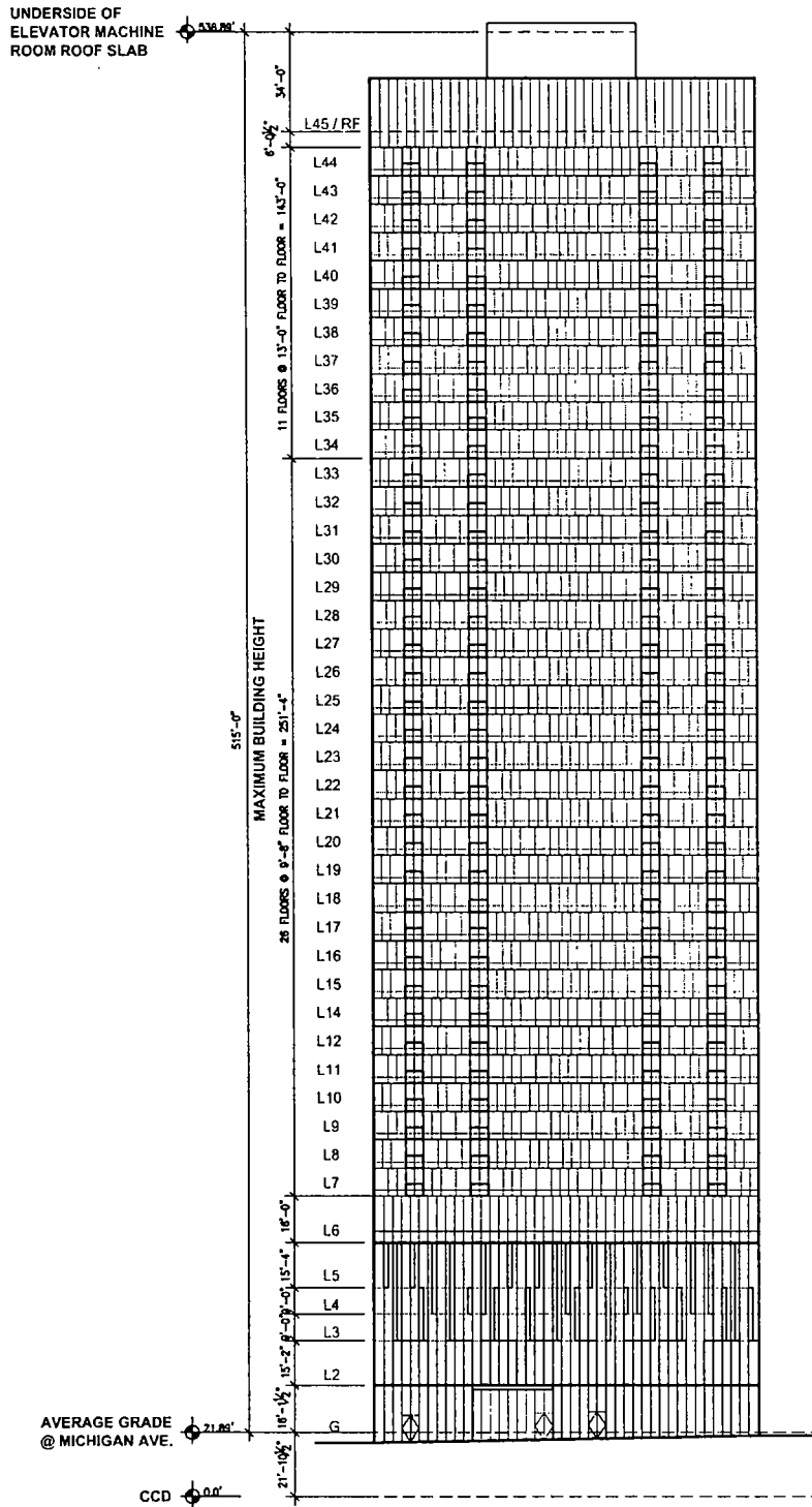
SOUTH BUILDING ELEVATION Scale: N.T.S.
