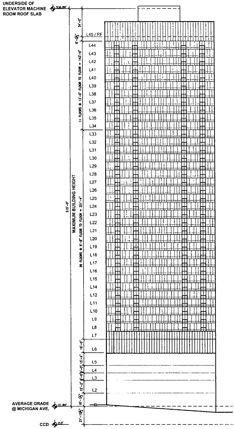
NORTH BUILDING ELEVATION Scale: N.T.S.
