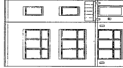
3926 S. Calumet Ave ELEVATION TYPE 'D'
