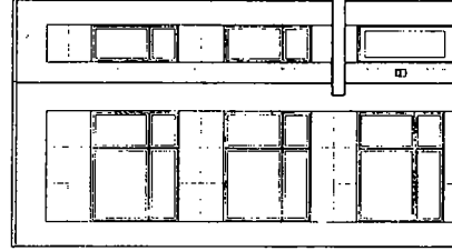
3528 S. Calumet Ave ELEVATION TYPE 'C'
