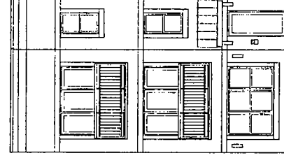
3922 S. Calumet Ave ELEVATION TYPE 'B'
