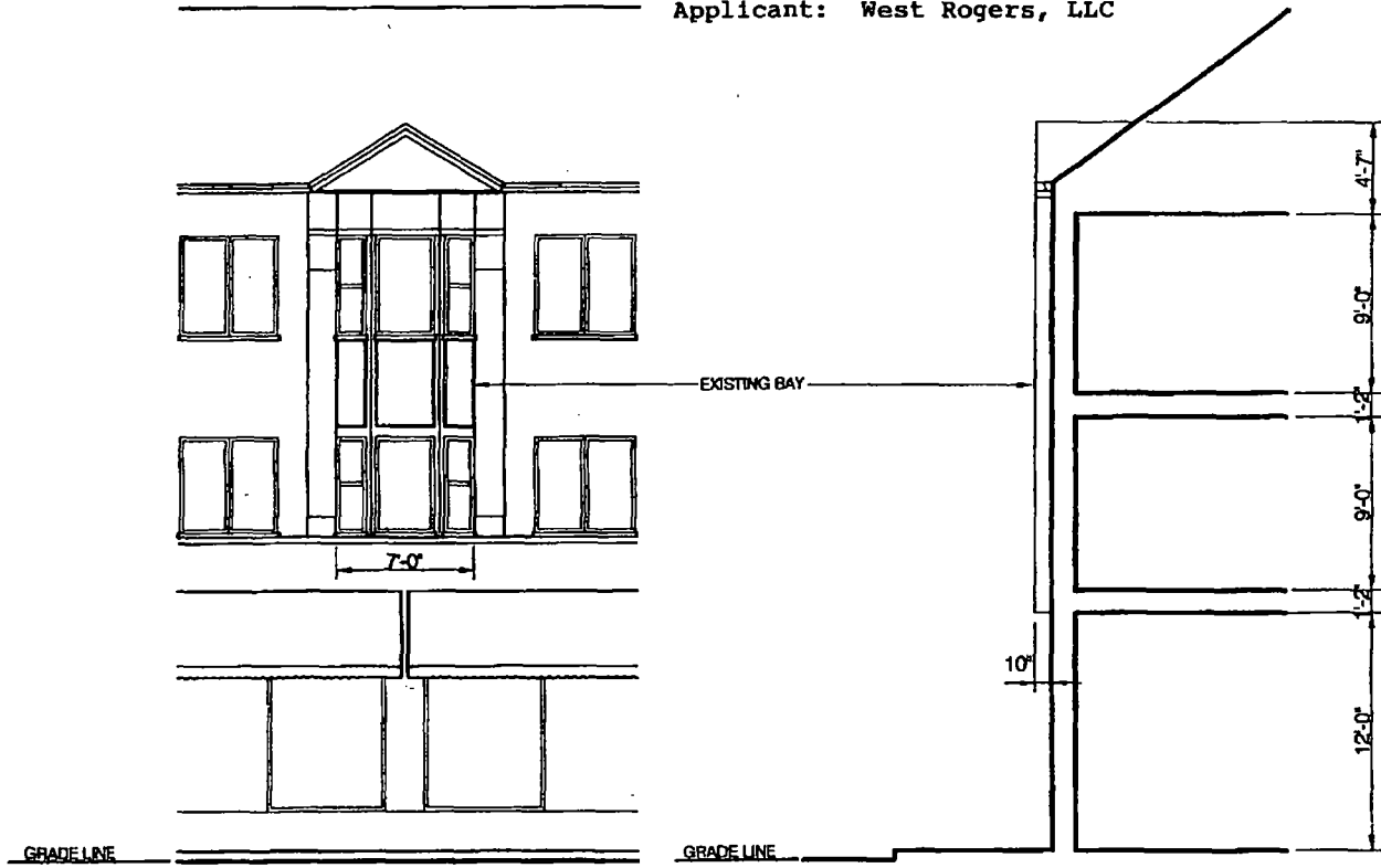
ELEVATION
