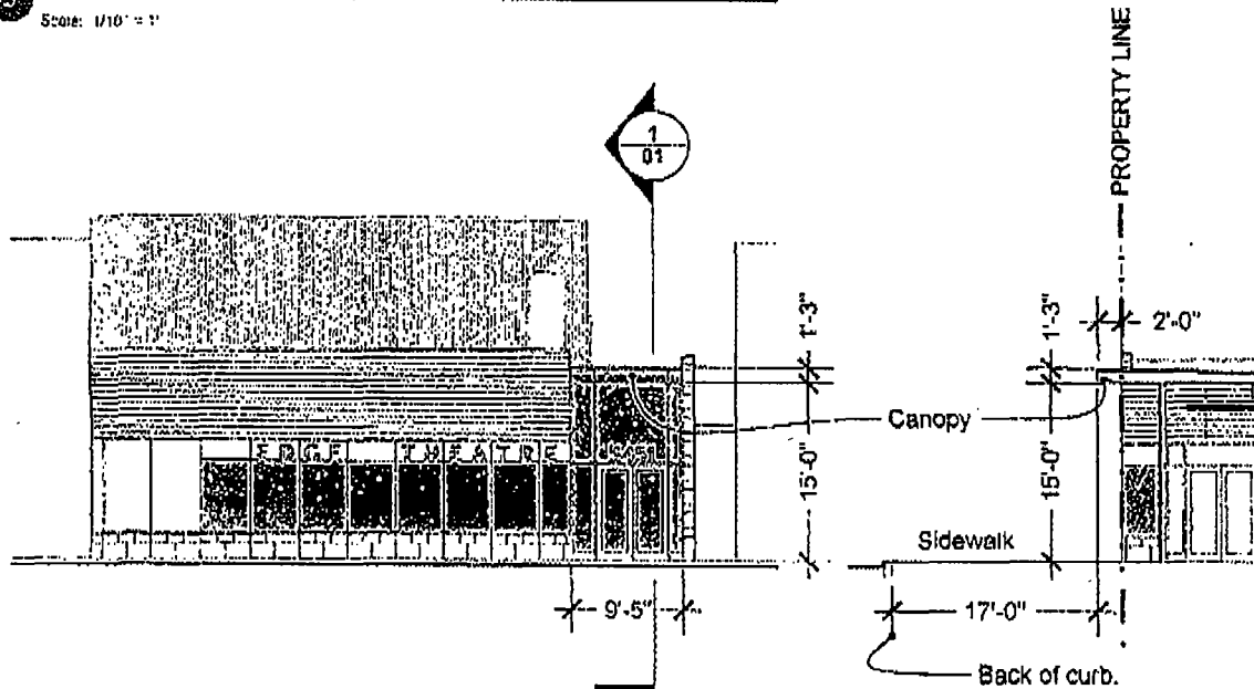
Elevation Scale: 1/16" = 1'
