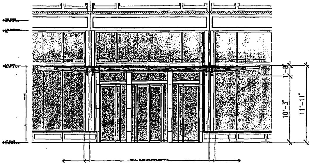
2 CANOPY ELEVATION SCALE: 1/8" = 1'-0"
