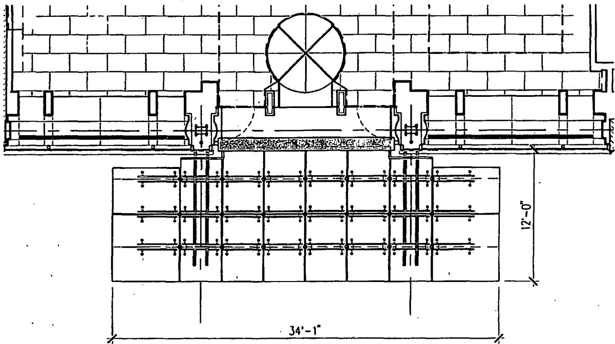
2 CANOPY ELEVATION SCALE: 1/8" = 1'-0"
