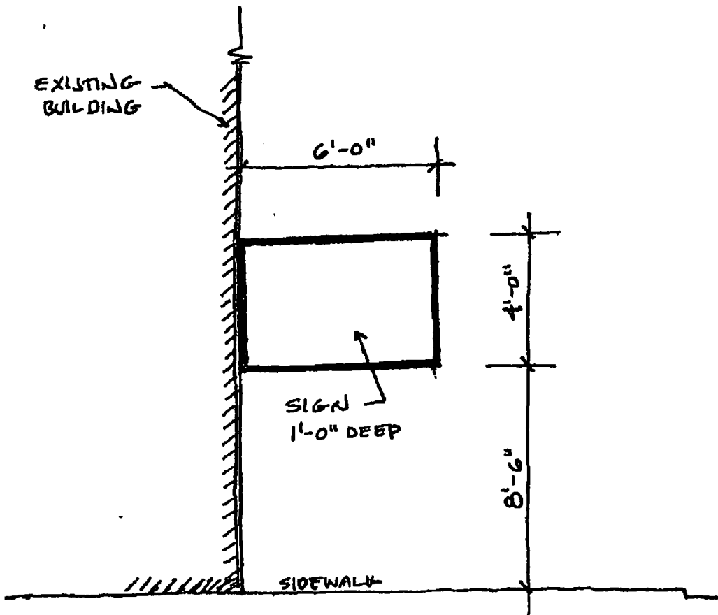
⊙ SIGN SIDE ELEVATION N.T.S.
