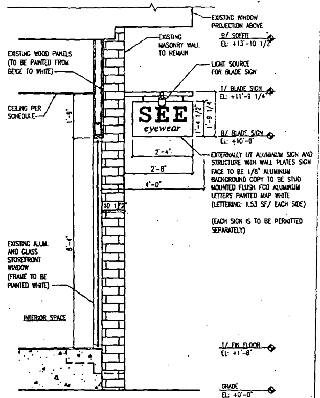
F11 SECTION @ STOREFRONT SCALE: 3/8" = 1'-0"
