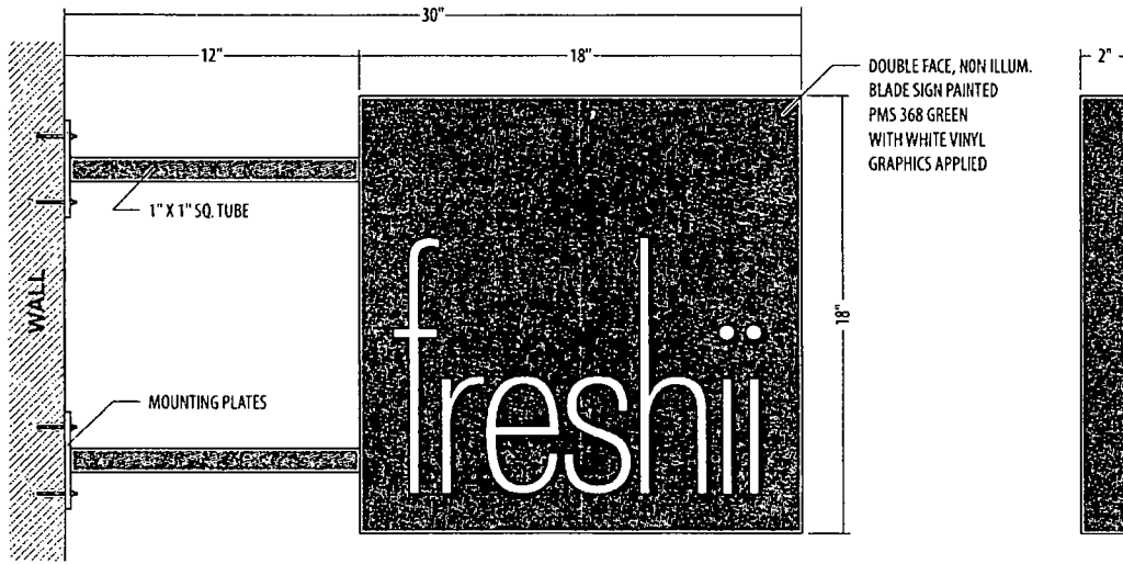
FRONT VIEW SCALE: 3"=1'-0"
