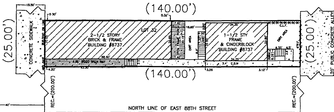
SCALE: 1"=20'
