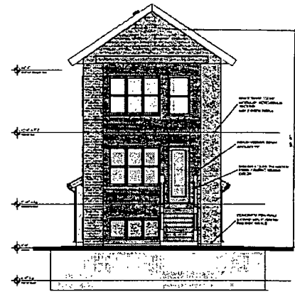
C NORTH ELEVATION SCALE: 1/8" = 1'-0"
