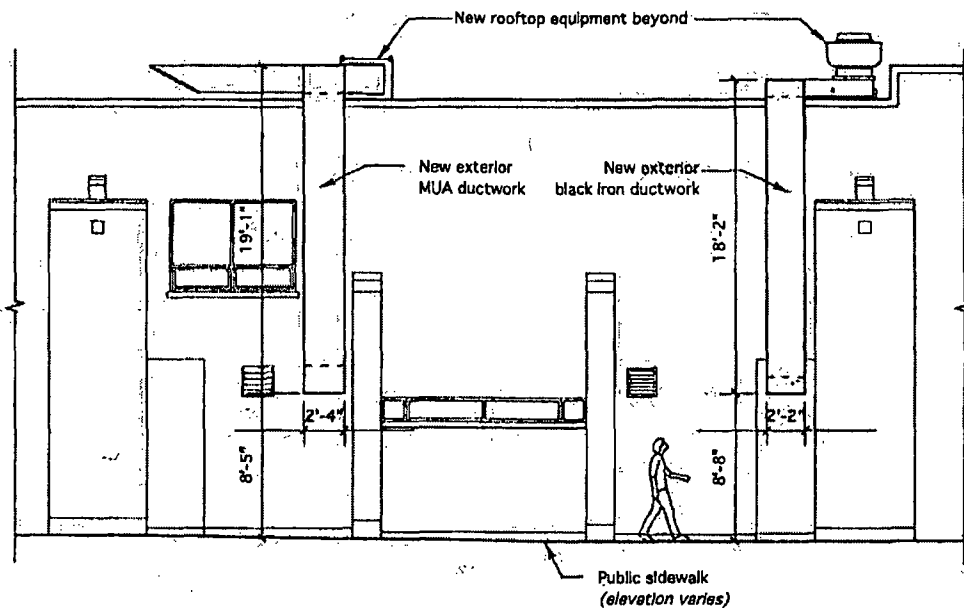
A. EXTERIOR ELEVATION (PARTIAL)
