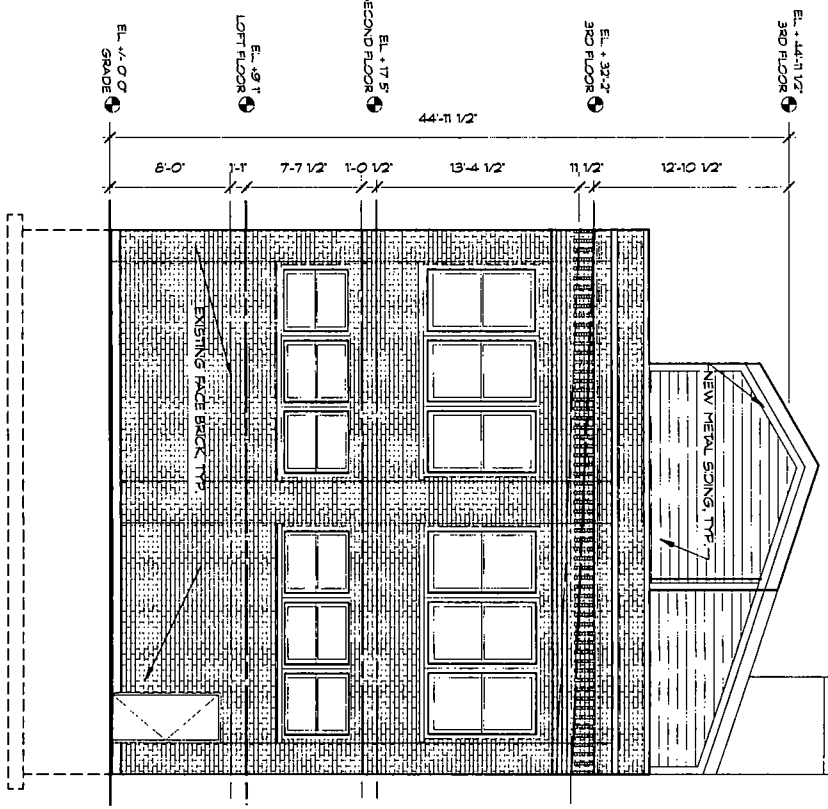
NEW WEST ELEVATION SCALE: 1/8" = 1'-0"
