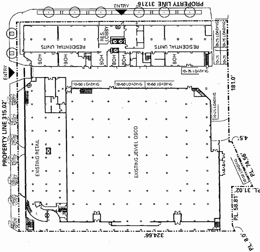
SITE PLAN (SUBAREA A) SCALE: 1/64" = 1'-0"
