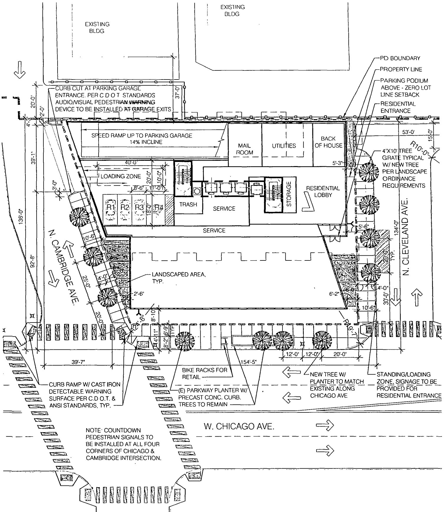
SITE /LANDSCAPE PLAN
