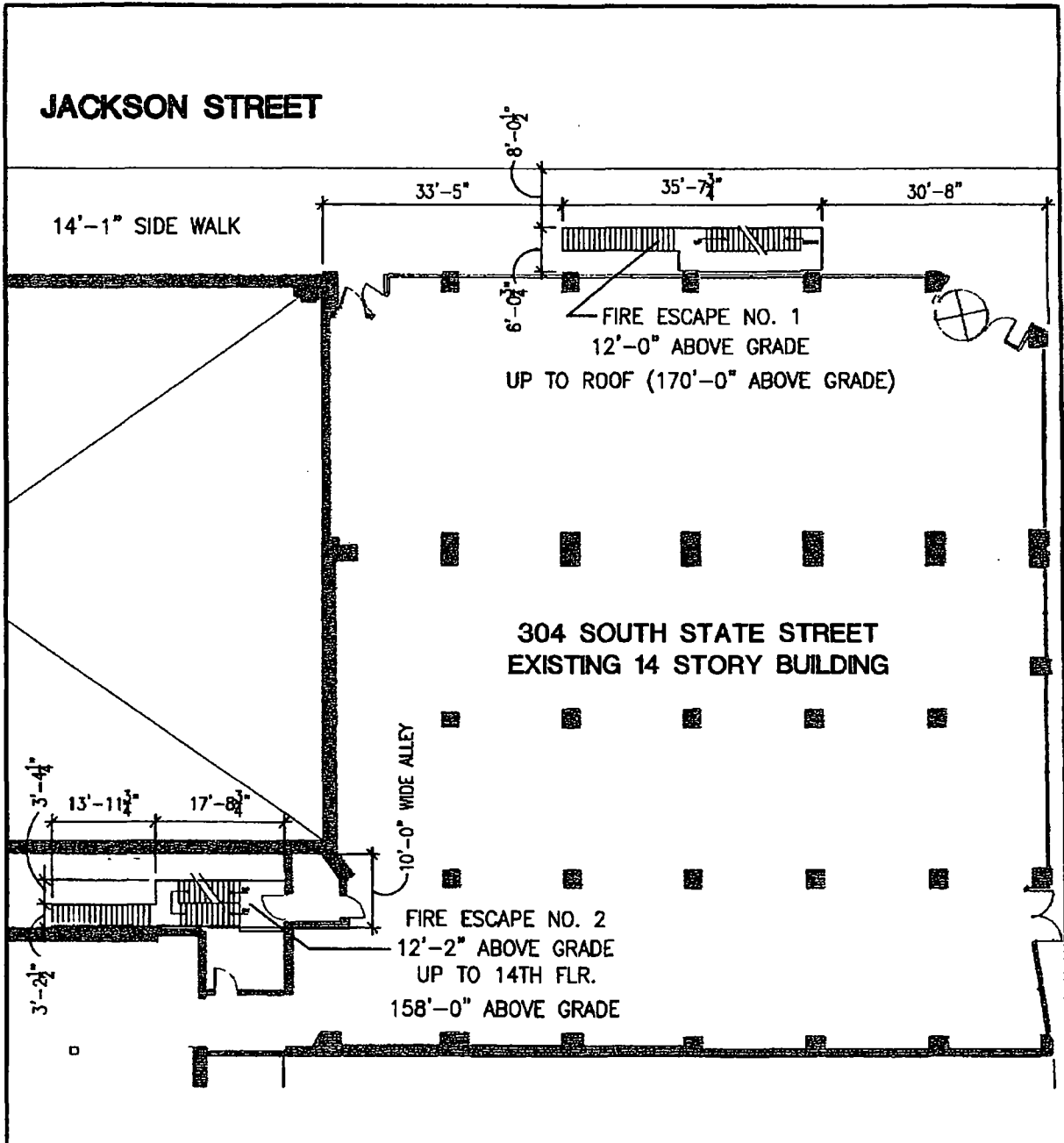
1 FIRE ESCAPE PLAN ASK-1 SCALE: 1" = 20'-0"
