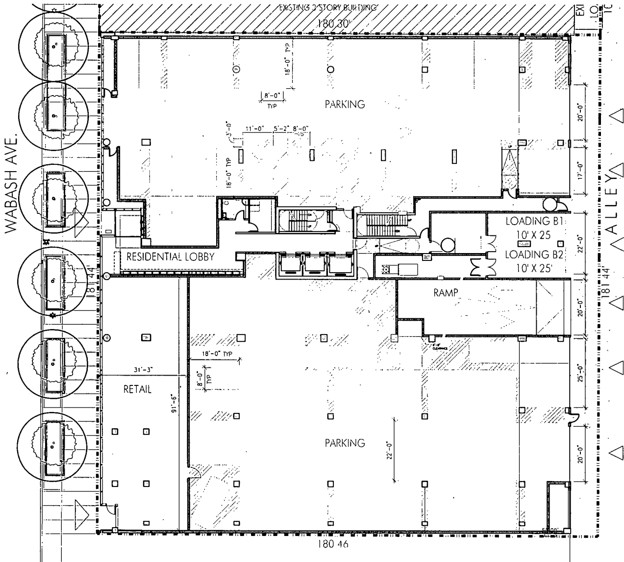
SITE PLAN (SUBAREA B)
