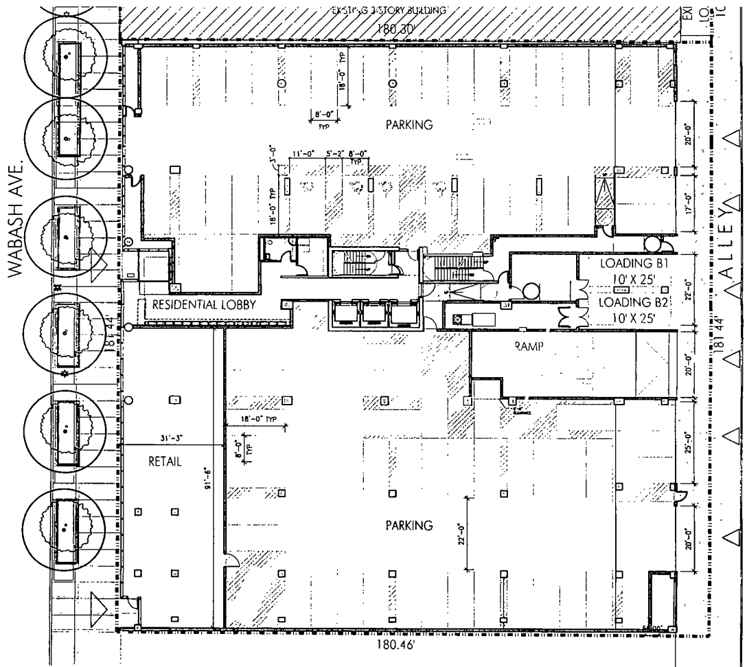
SITE PLAN (SUBAREA B)
