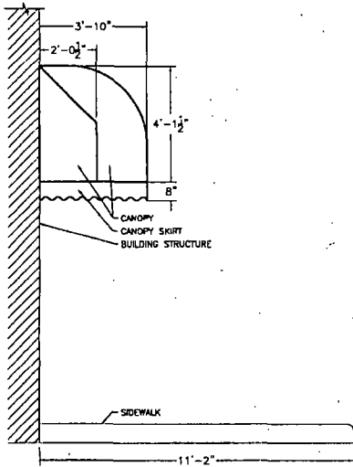
WEST ELEVATION N.T.S
