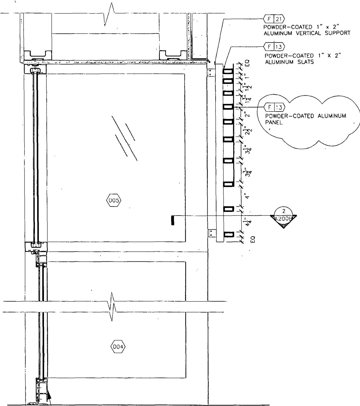
3 SECTION SCALE: 3/4" = 1'-0"
