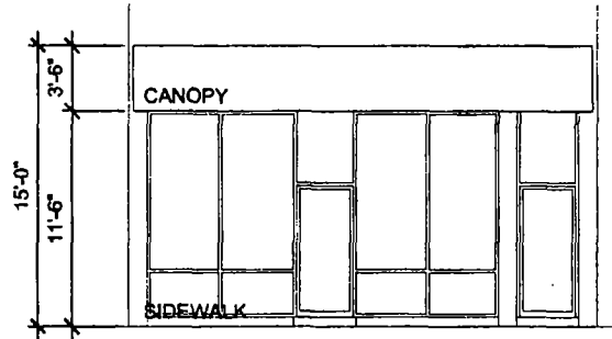
2 WEST ELEVATION SCALE: 1/8" = 1'-0"
