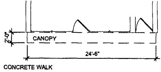
3 PLAN SCALE: 1/8" = 1'-0"
