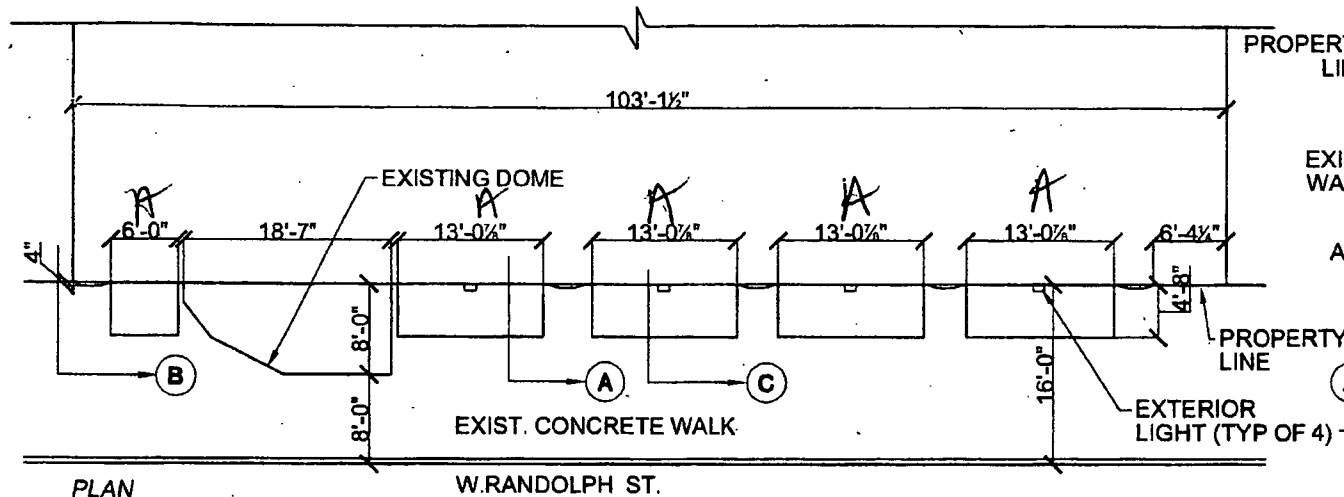
PLAN SCALE: 1/16" = 1'-0"
