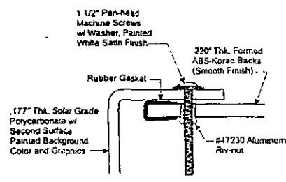
Face Mounting Detail Scale: N.T.S.
