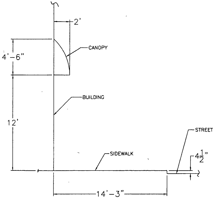
SIDE ELEVATION 9044-46 1/2 S. ASHLAND
