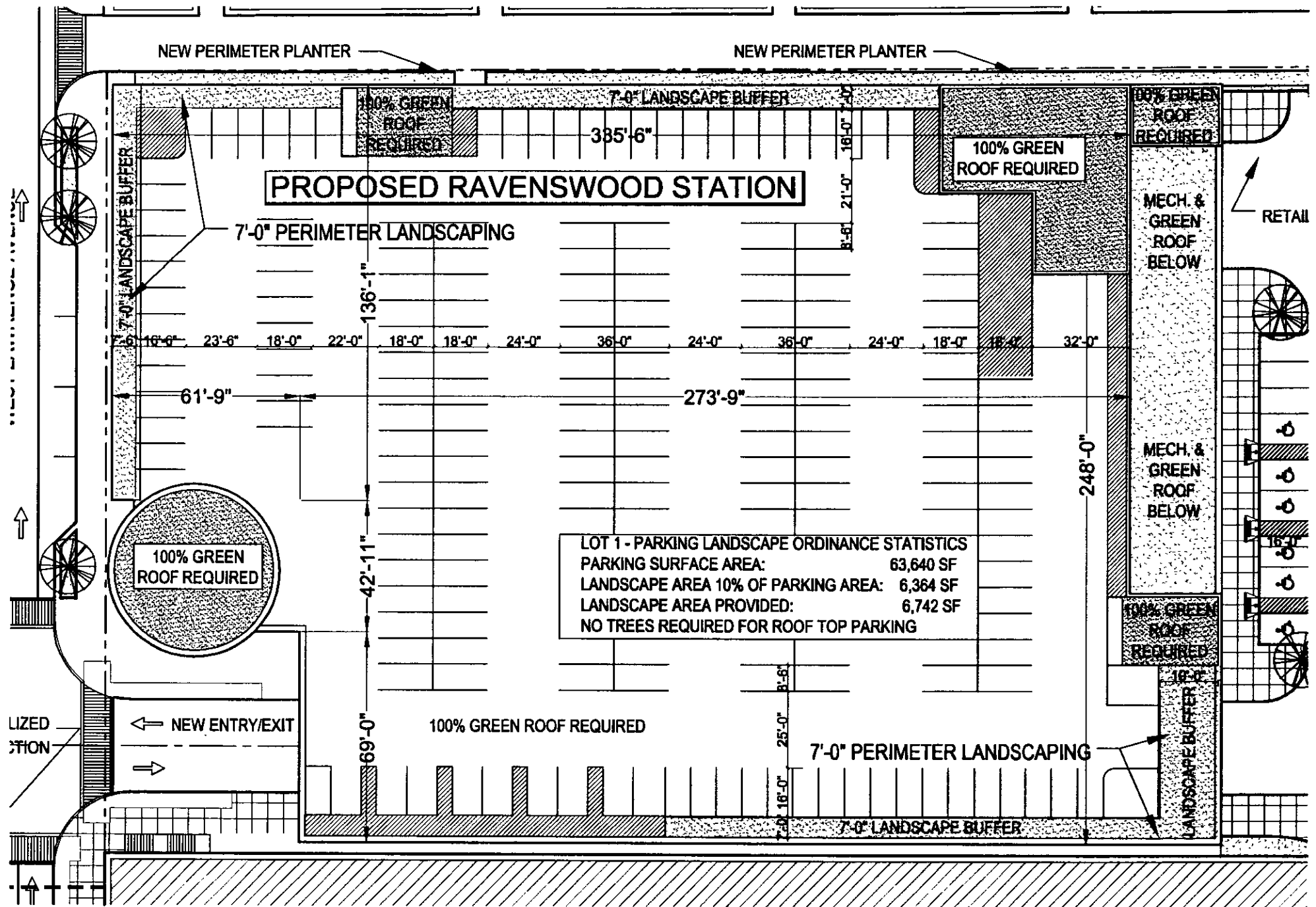
E3. Roof Plan
