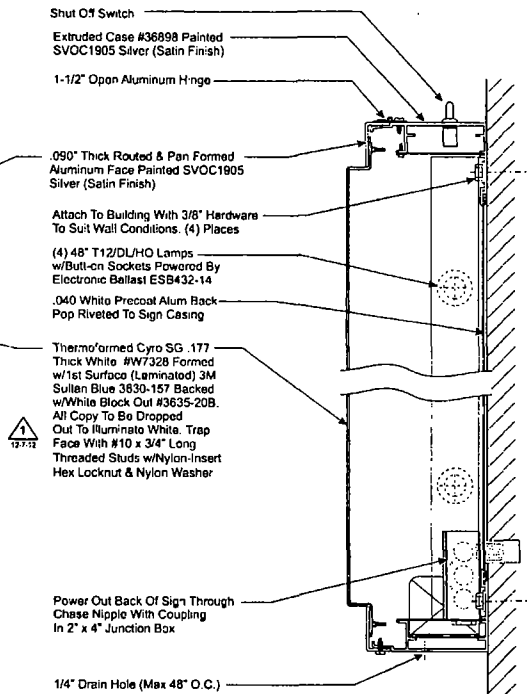
SECTION SCALE: 3" = 1'-0"
