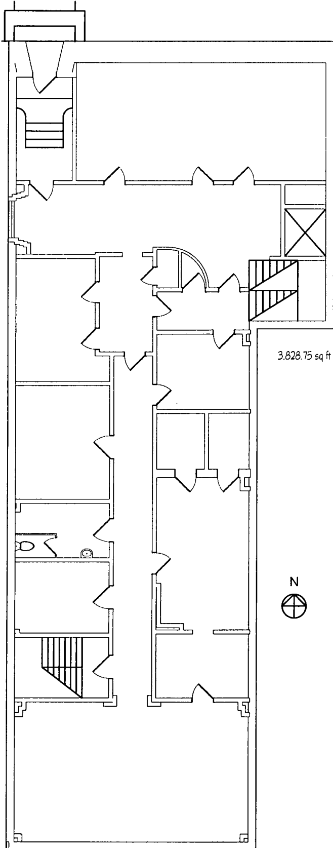
1. First Floor SCALE: 1/8" = 1'-0"
