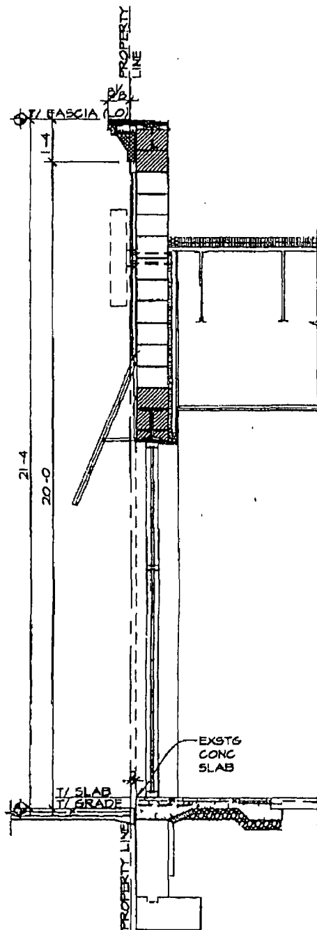
SECTION @ CORNICE 1 SCALE: 9/8" = 1'-0"
