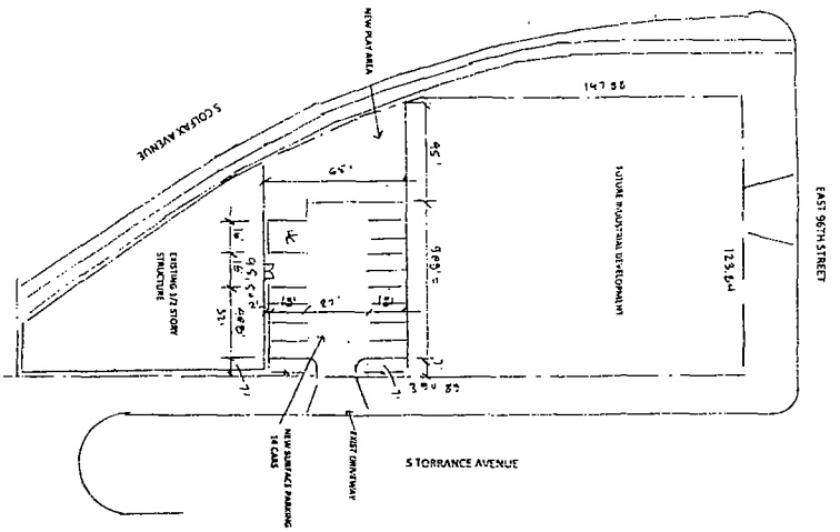
1 SITE PLAN 1"=12'
