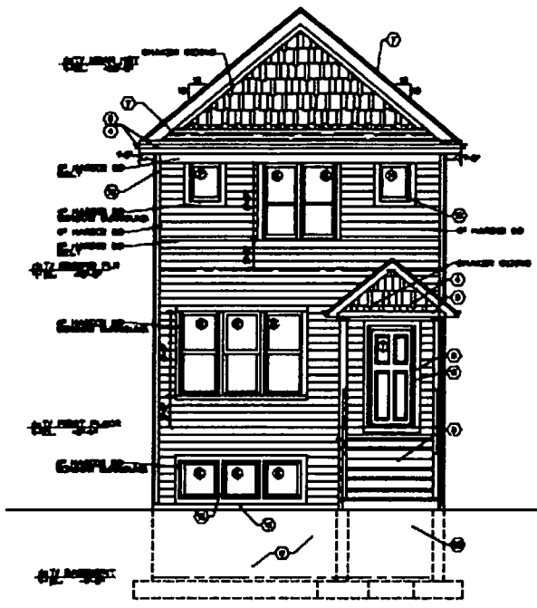
4 FRONT ELEVATION (SCALE) 1/8" = 1'-0"
