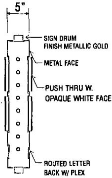
D/F ILLUM. SIGN SECTION SCALE: 1 1/2" = 1'-0"
