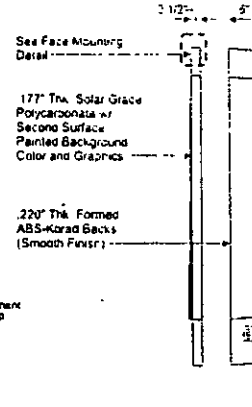
Side View Scale: N.T.S.
