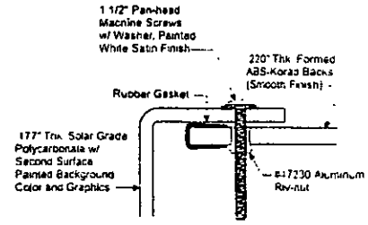
Face Mounting Detail Scale: N.T.S.
