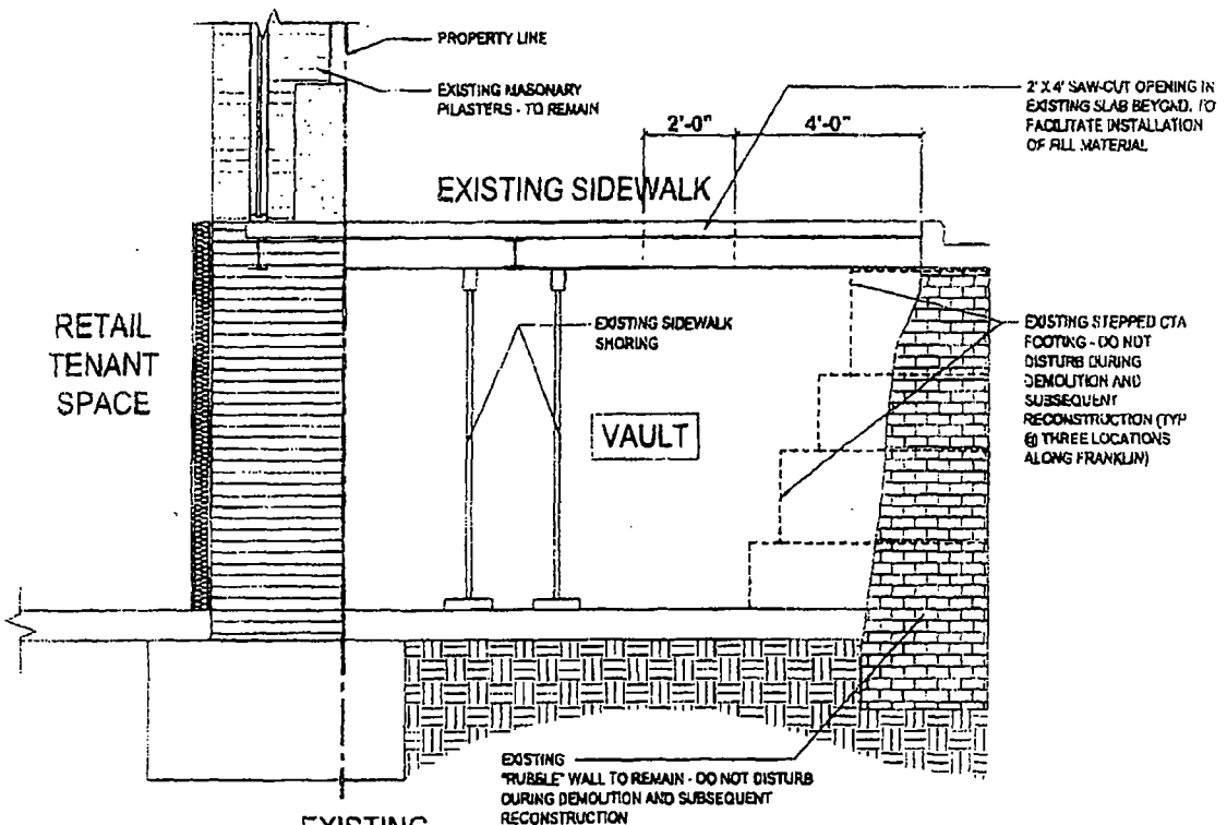
1 EXISTING SIDEWALK SECTION ASO SCALE: 3/8" = 1'-0"
