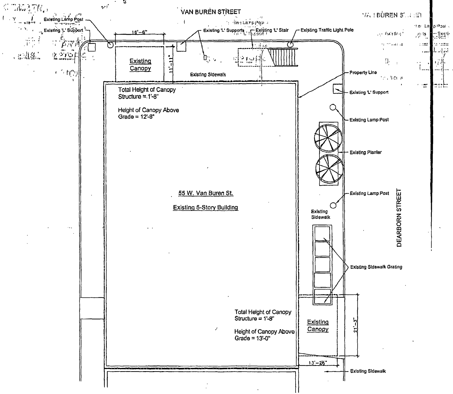
Existing Site Plan - 55 W. Van Buren Street
