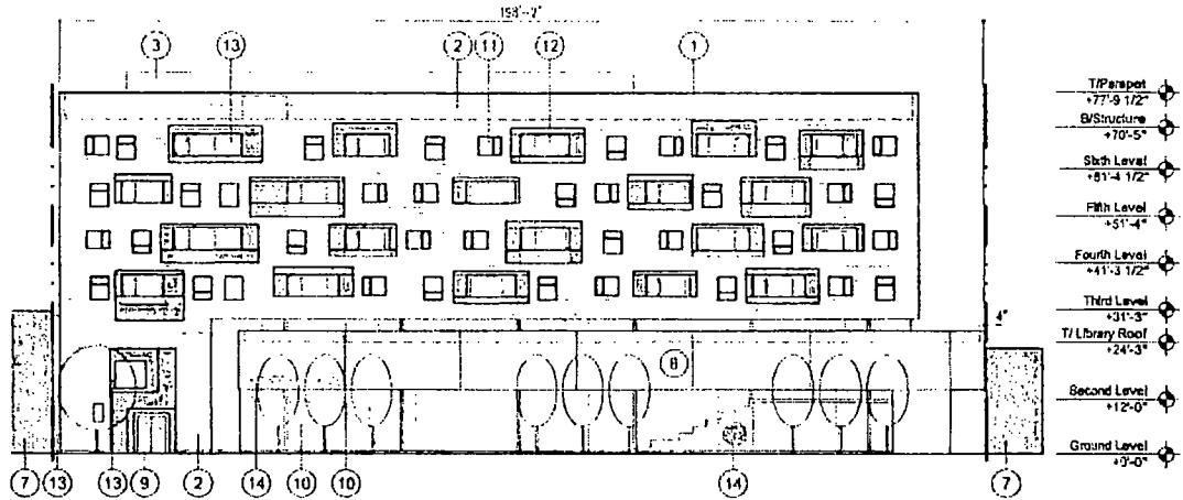
A. EAST ELEVATION
