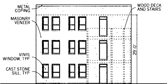
G2 - Rear Elevation
