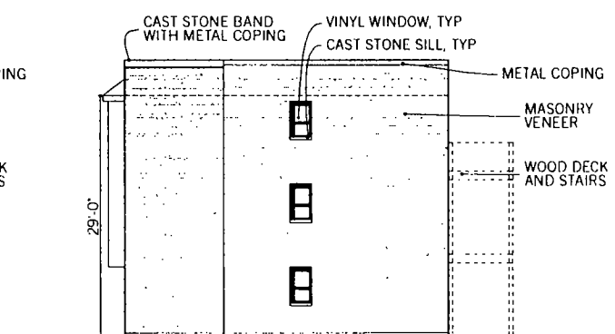
G2 - Side Elevation
