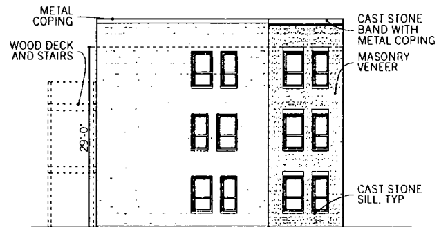
G2 - Side Elevation
