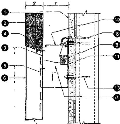
Section @ LED Logo Raceway Scale: N.T.S.
