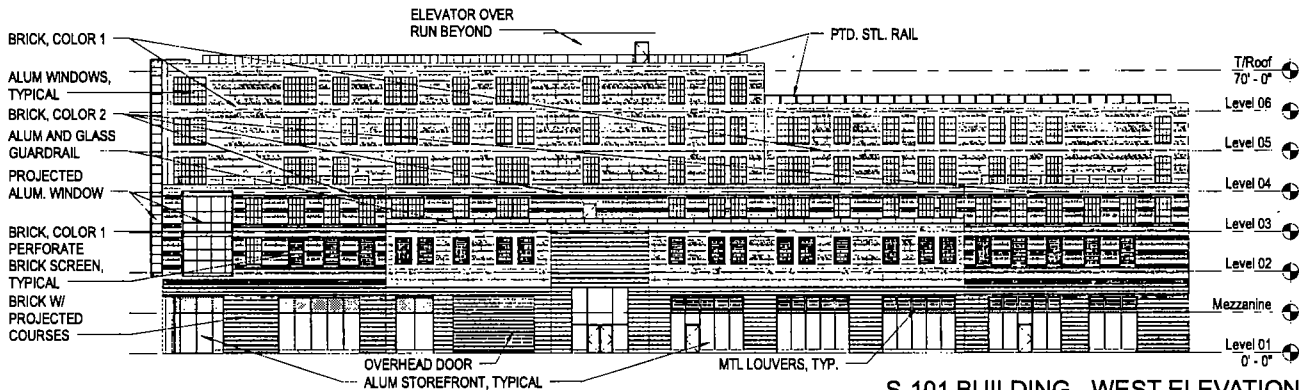
S-101 BUILDING - WEST ELEVATION Scale: N.T.S.
