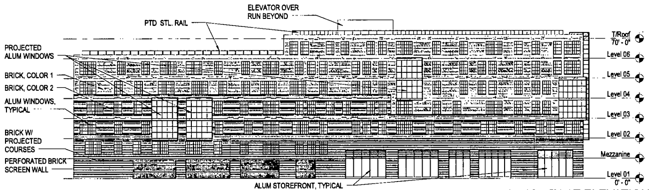
S-101 BUILDING - EAST ELEVATION Scale: N.T.S.
