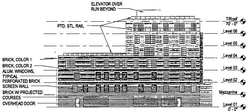
S-101 BUILDING - SOUTH ELEVATION Scale: N.T.S.
