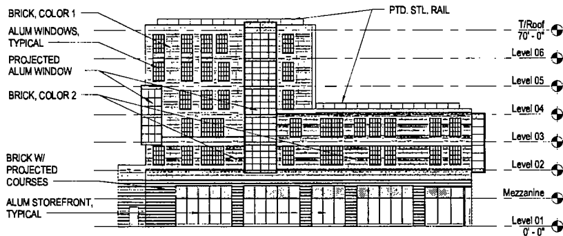
S-101 BUILDING - NORTH ELEVATION Scale: N.T.S.
