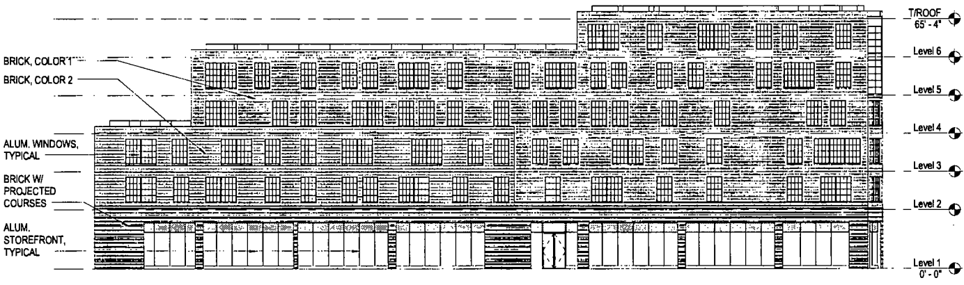
N-101 BUILDING - SOUTH ELEVATION Scale: N.T.S.
