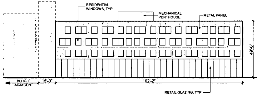
4 Bldg E - West SCALE: 1" = 50'
