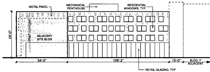
3 Bldg E - East SCALE: 1" = 50'
