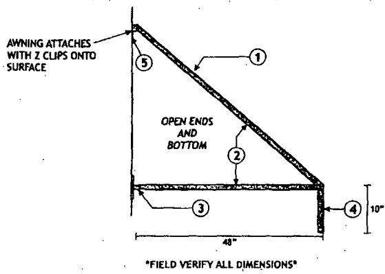
AWNING - SECTION Scale: N.T.S.
