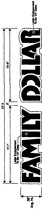
Front View - 36" Linear Cloud Scale: 3/8" = 1'-0"
