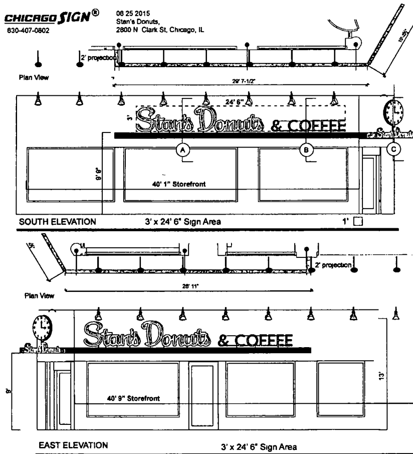
SE Elevation
