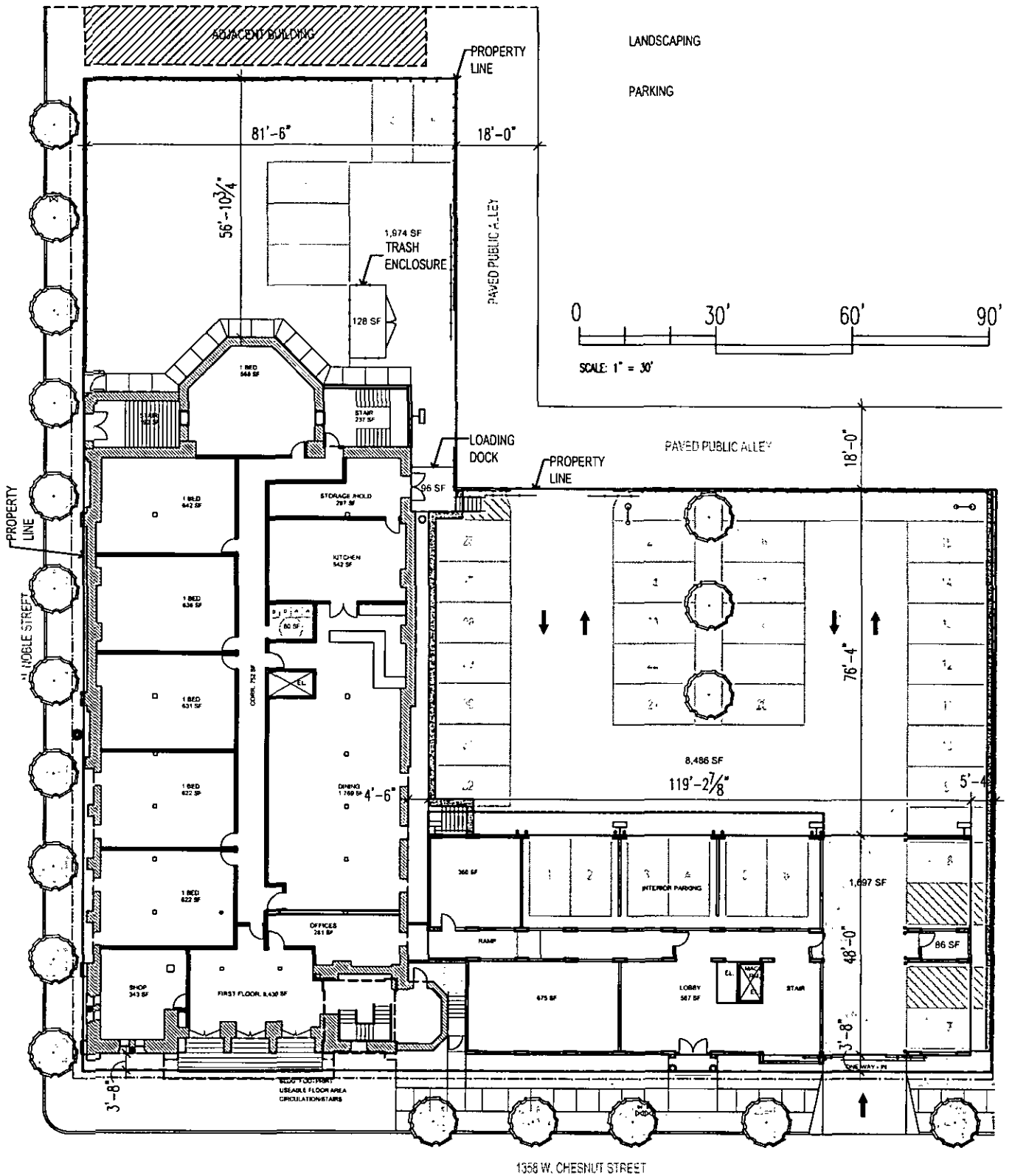
Site Plan Level 01
