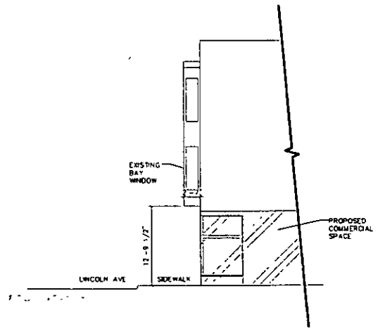
② SOUTH ELEVATION N.T.S.
