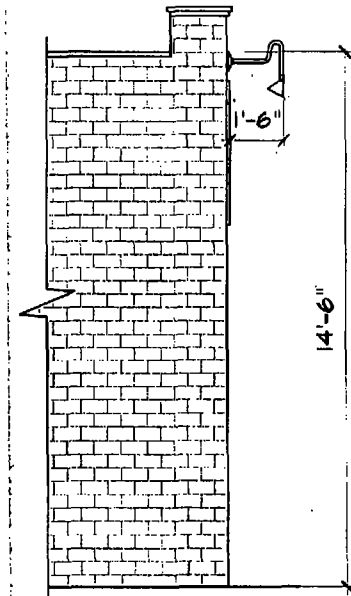
SIDE ELEVATION SCALE: 1/4" = 1'-0"
