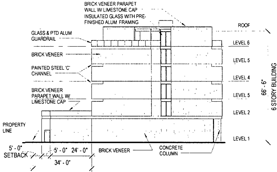
EAST BUILDING ELEVATION Scale: N.T.S.
