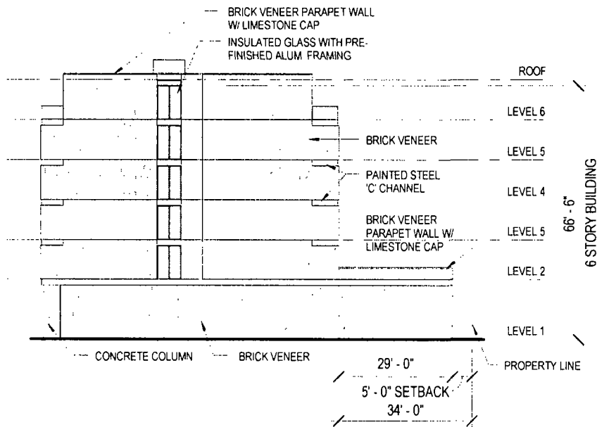
WEST BUILDING ELEVATION Scale: N.T.S.
