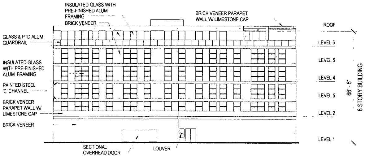
SOUTH BUILDING ELEVATION Scale: N.T.S.
