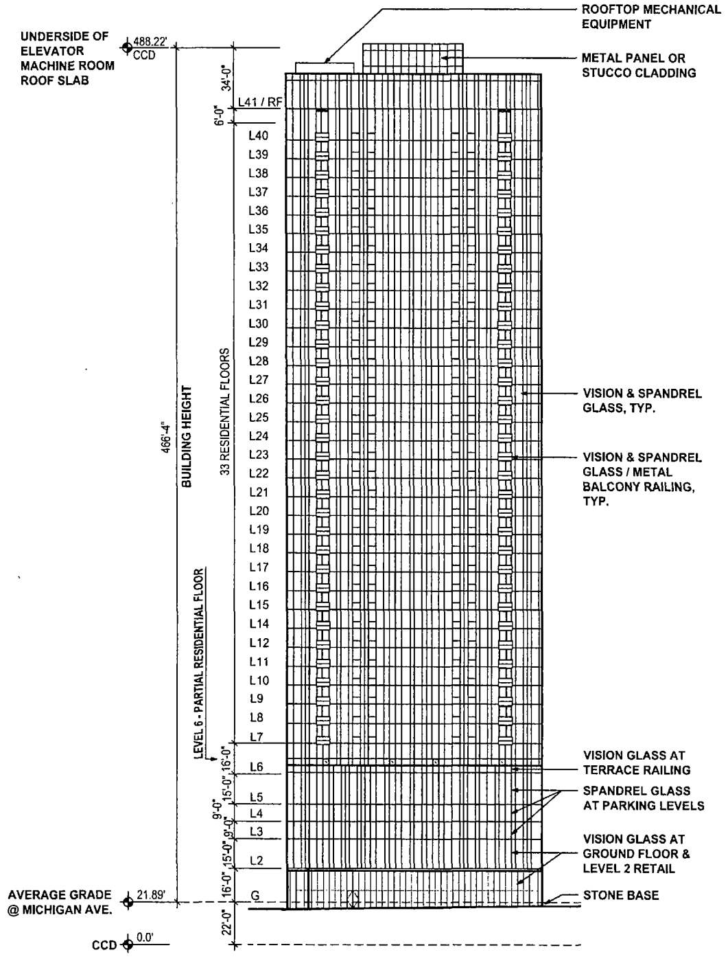
SOUTH BUILDING ELEVATION Scale: N.T.S.
