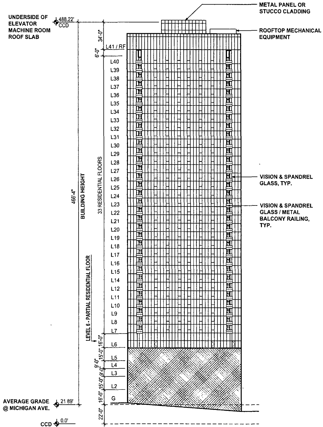
NORTH BUILDING ELEVATION Scale: N.T.S.
