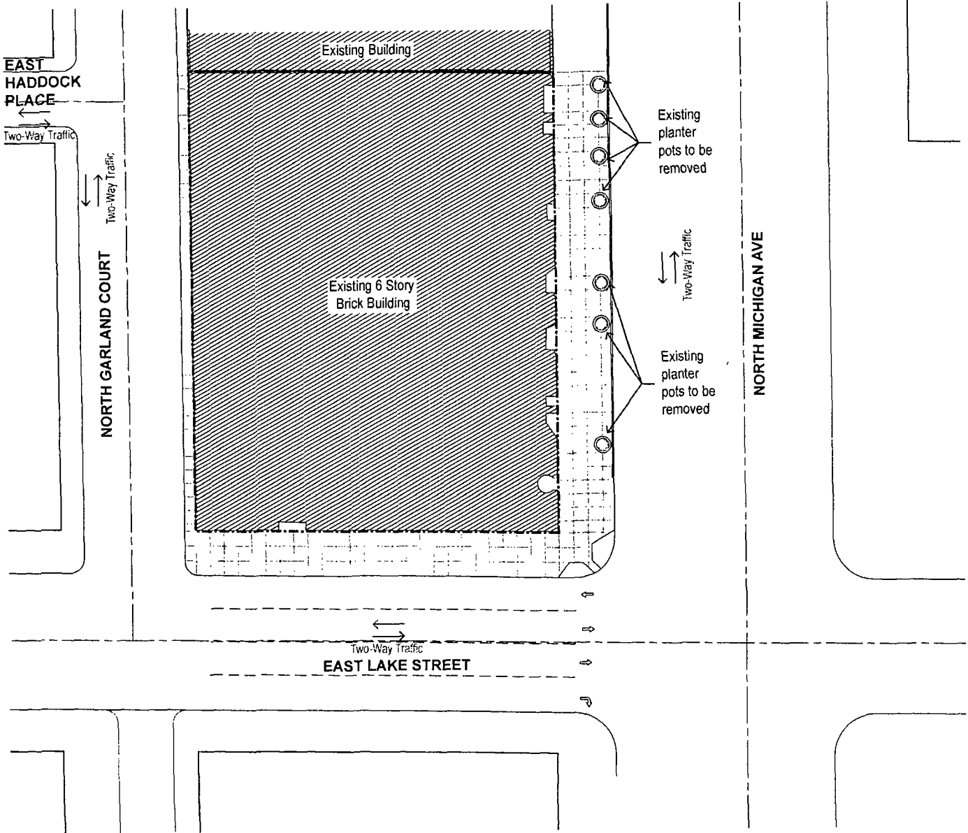
EXISTING SITE PLAN Scale: N.T.S.
