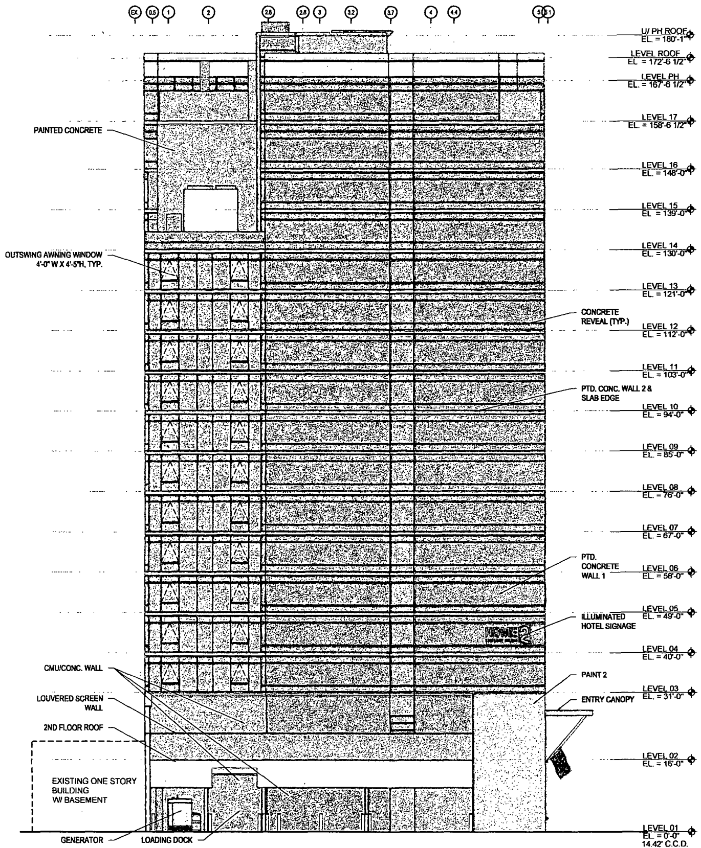
1 WEST ELEVATION (ALLEY) SCALE: N.T.S.
