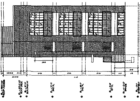
EAST ELEVATION SCALE: 1/8" = 1'-0"
