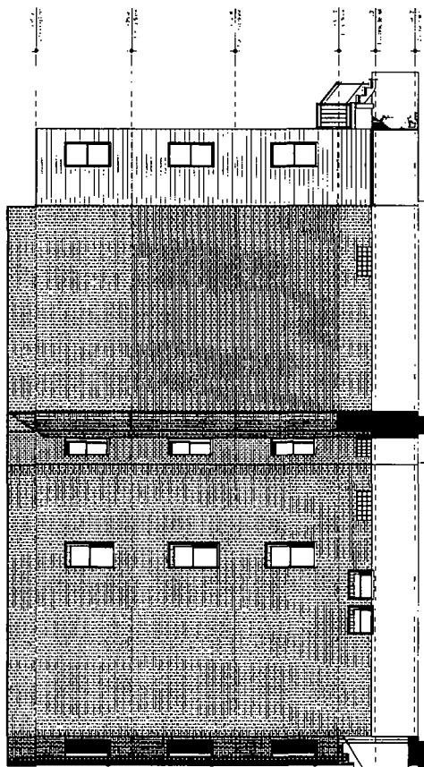
Right Elevation
