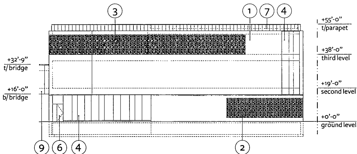
A. WEST ELEVATION - TCAC
