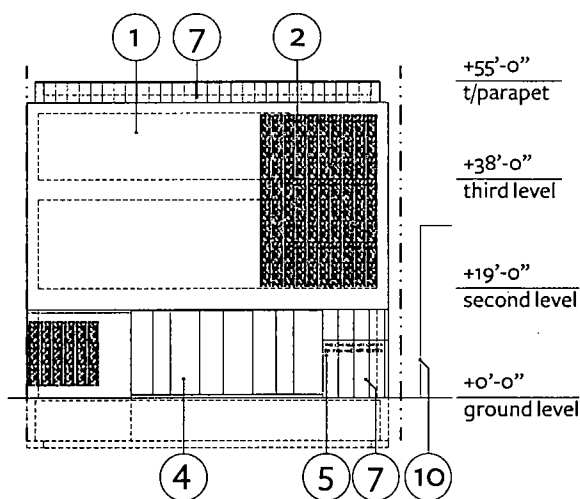
B. SOUTH ELEVATION - TCAC
