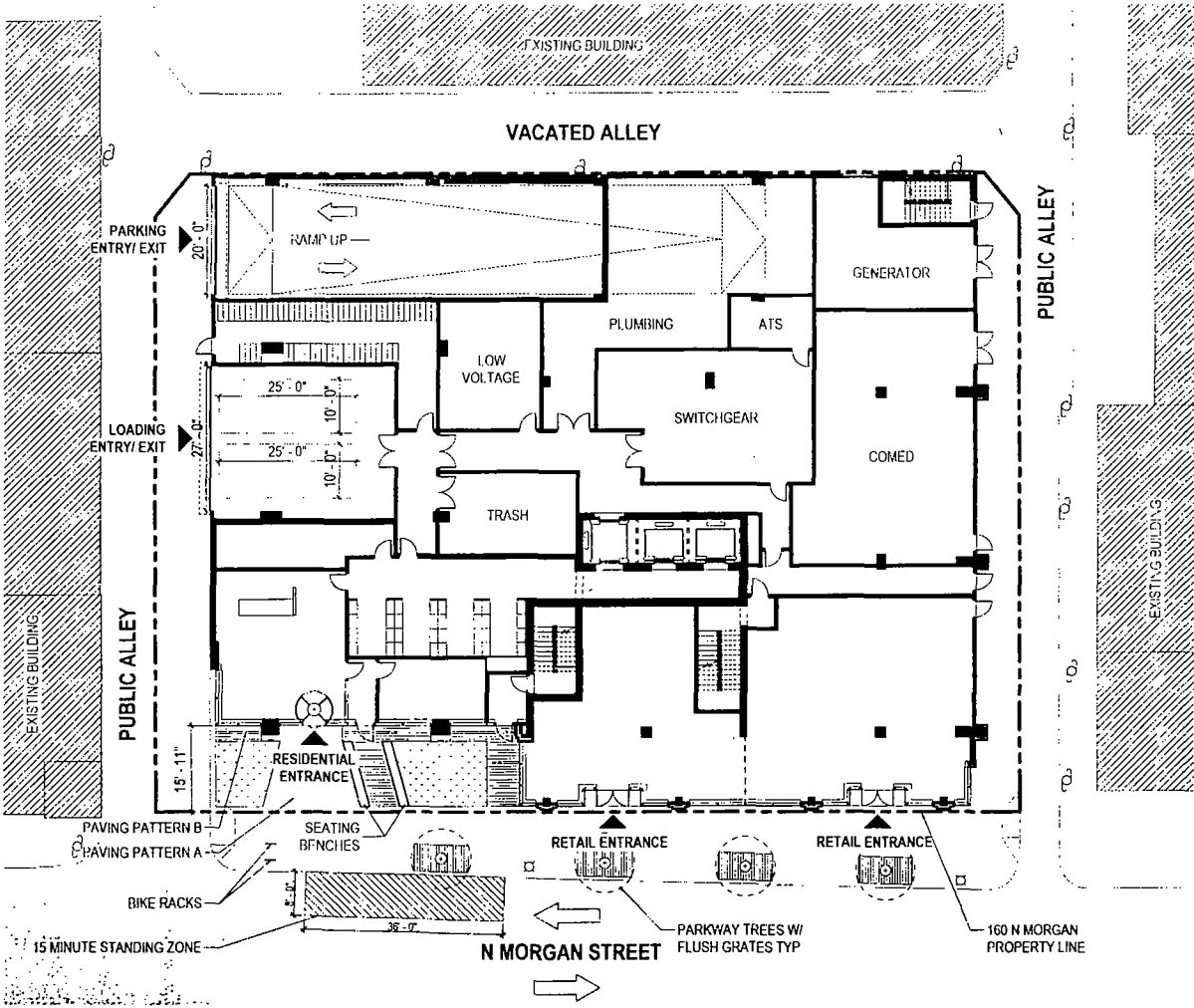
GROUND LEVEL PLAN Scale: N.T.S.
